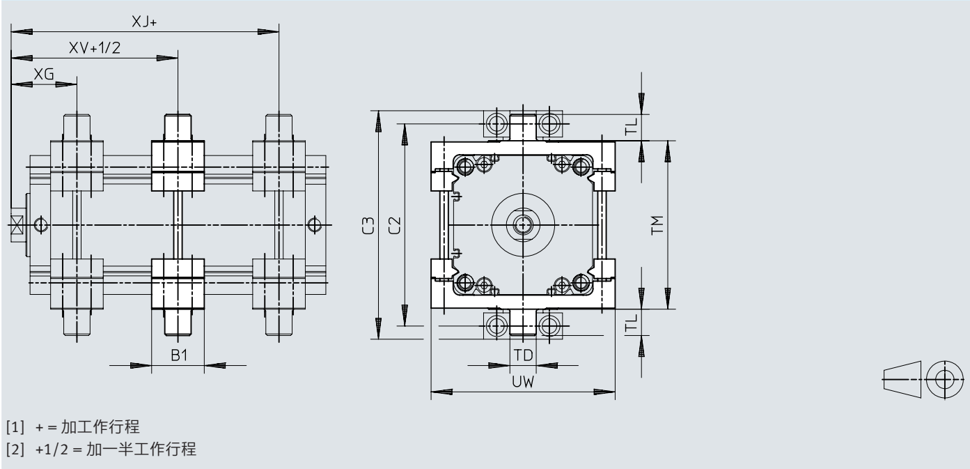
尺寸 – 耳轴安装件套件 DAMT-V7-125-A, 适用于缸径 125 mm
