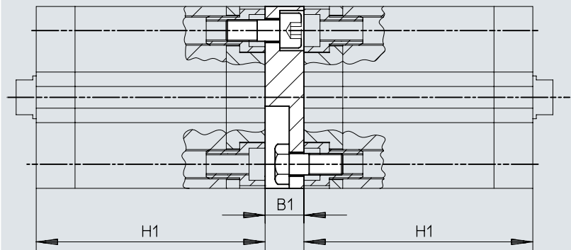
尺寸 – 多位置安装组件 DPVU，适用于缸径 12 ... 100 mm
