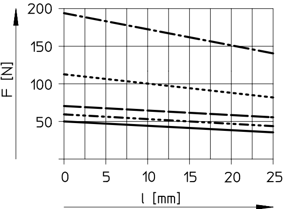
弹簧回复力 F 与冲程的关系 - AEVU
