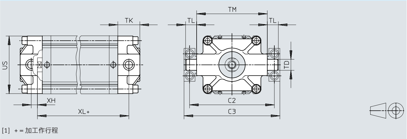
尺寸 – 耳轴安装件 ZNCF-125, 适用于缸径 125 mm
