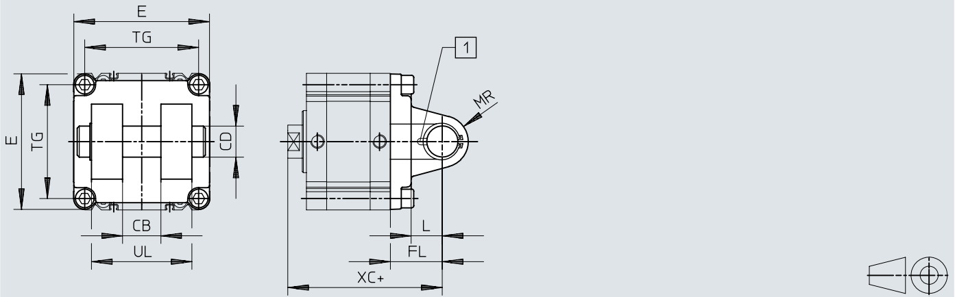
尺寸 – 双耳环安装件 SNC-125, 适用于缸径 125 mm
