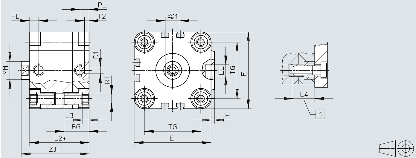
尺寸 – 基本型, 缸径 12 ... 100 mm
