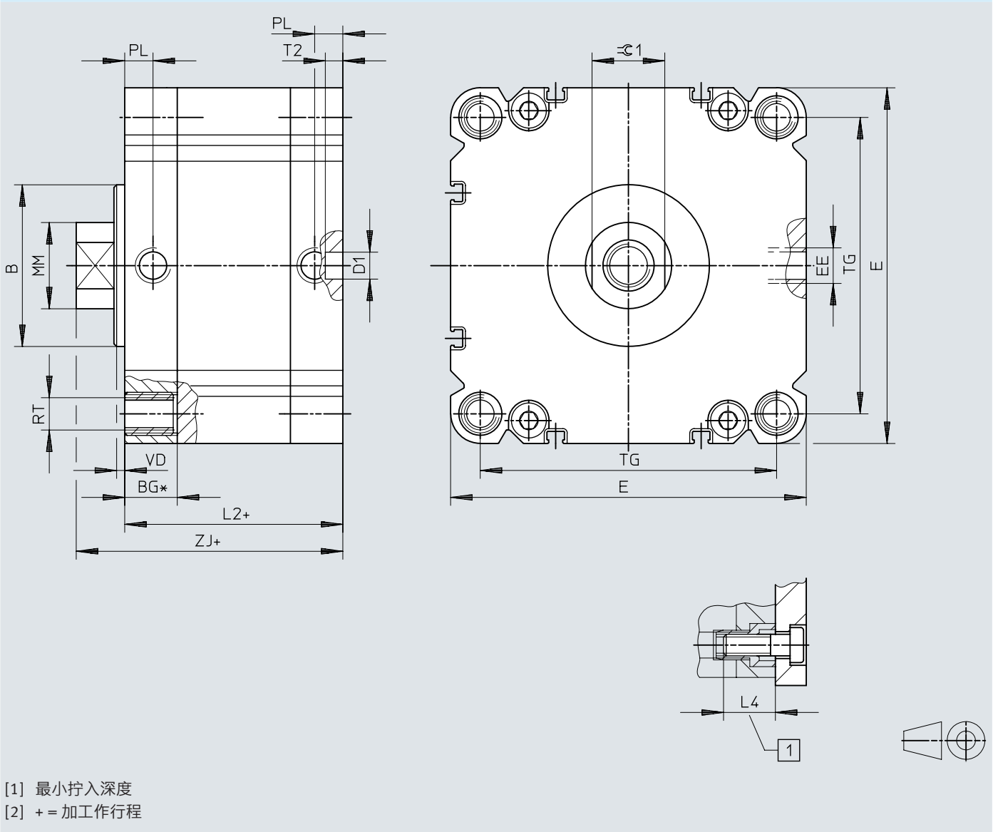
尺寸 - 基本型, 缸径 125 mm
