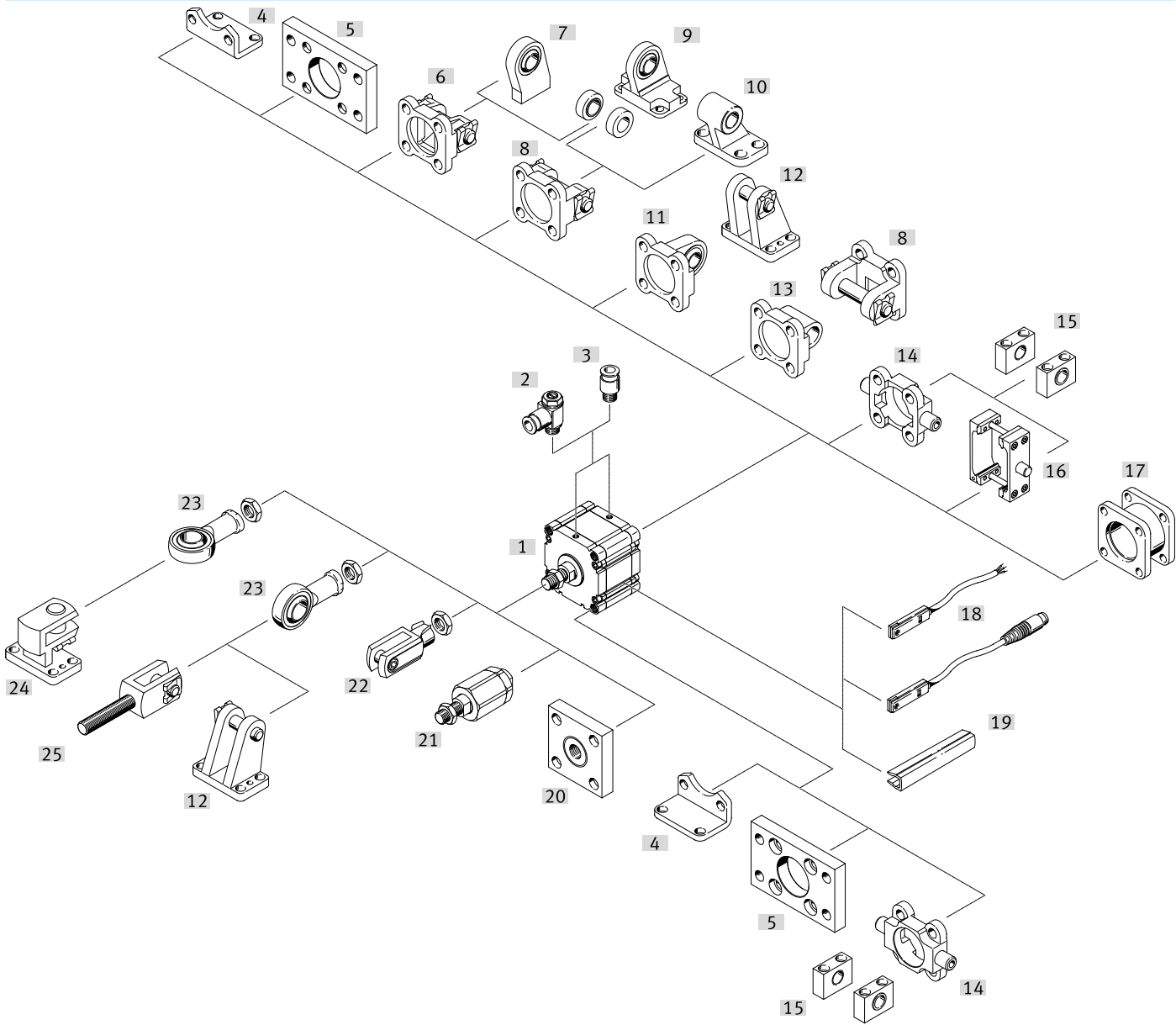
外围元件一览 ADVU-125
