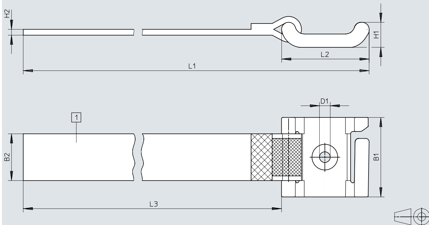
尺寸 - 气管支撑件 NPAW
