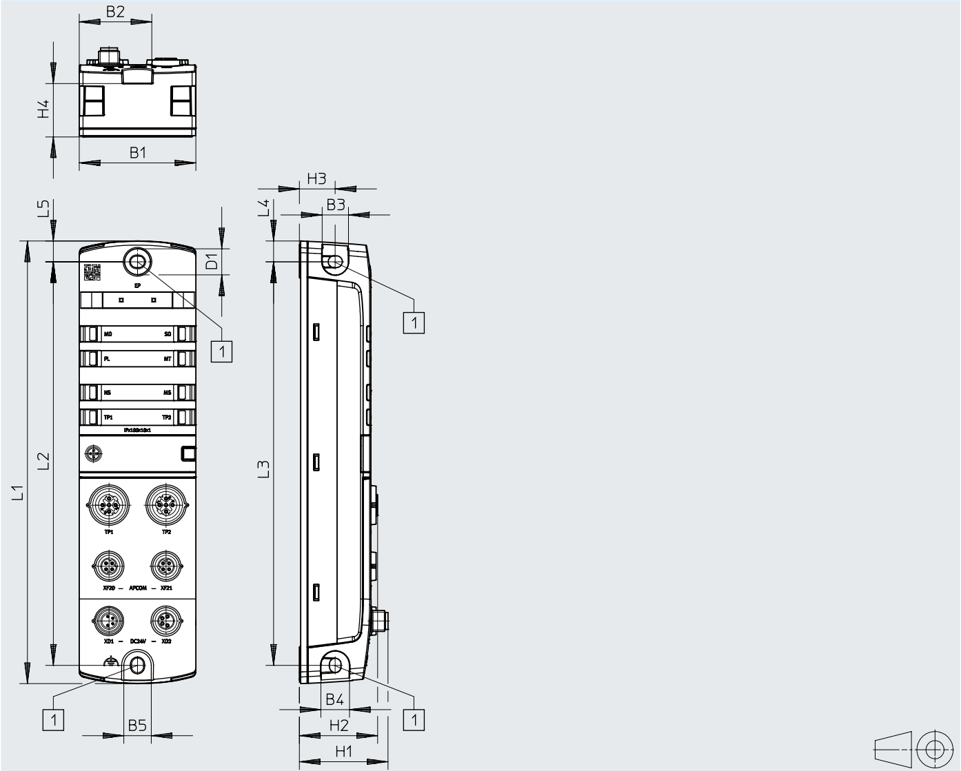
[1] 安装孔，用于 M4 螺丝
