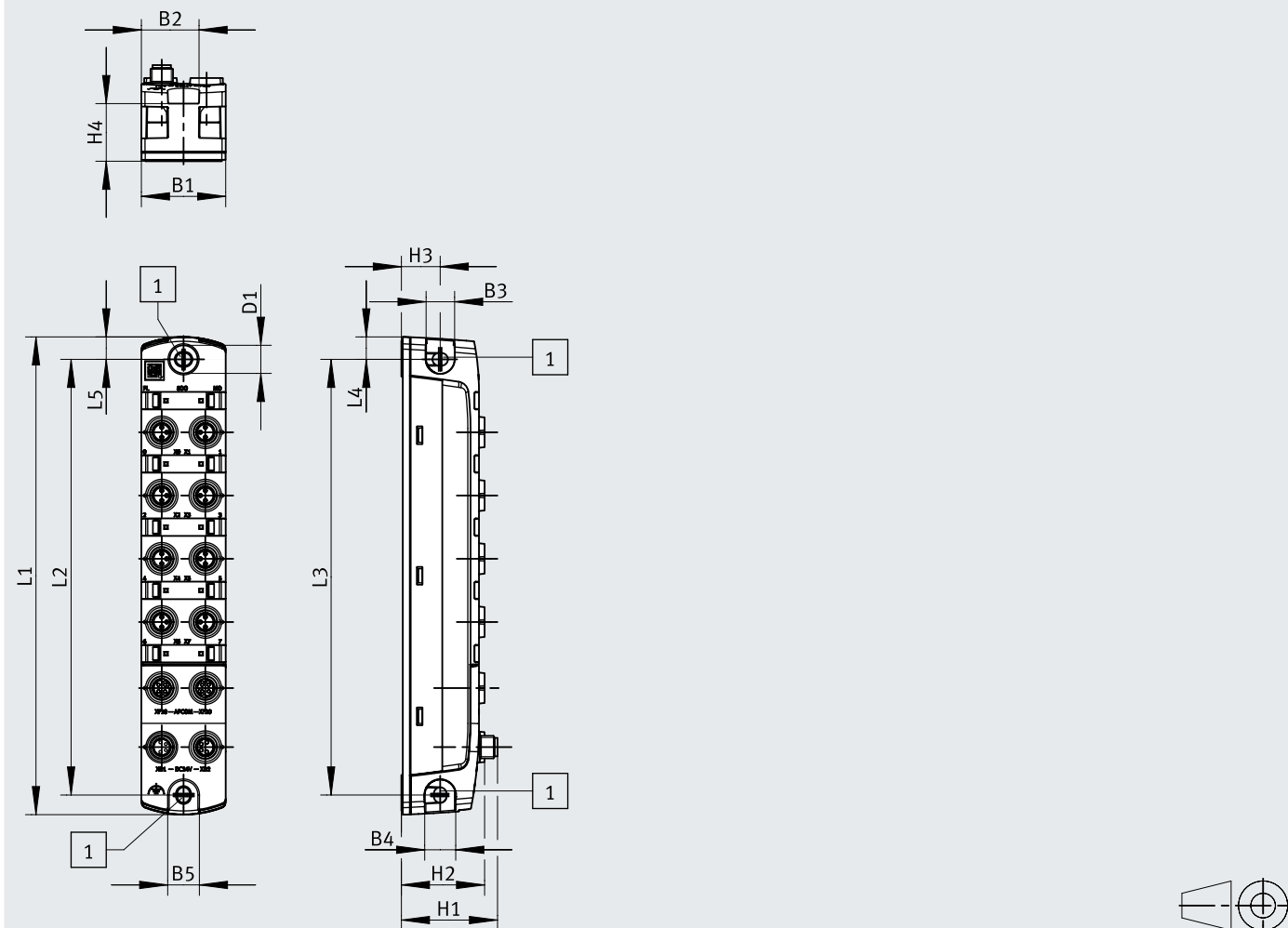
尺寸 – CPX-AP-I-8DO-M8-3P
