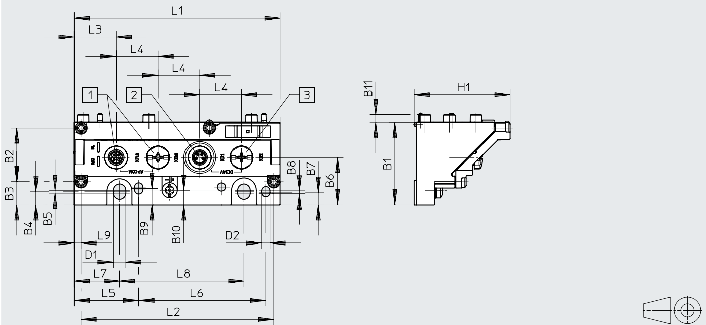
[1] 插座 M8x1, D编码 [2] 插头 M8x1, A编码 [3] 插座 M8x1, A编码
