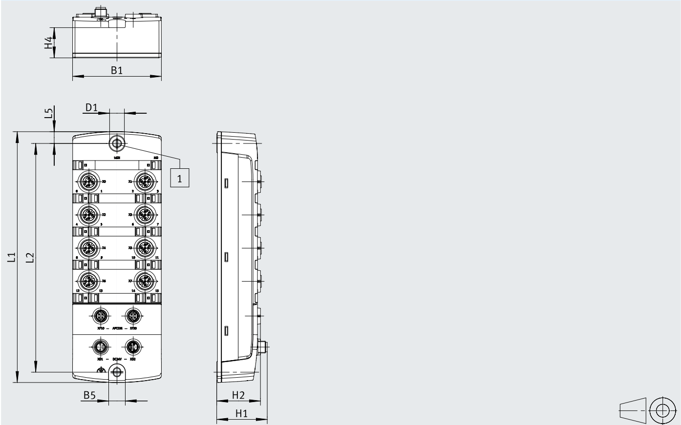
尺寸 - CPX-AP-I-16DI-M12-5P
