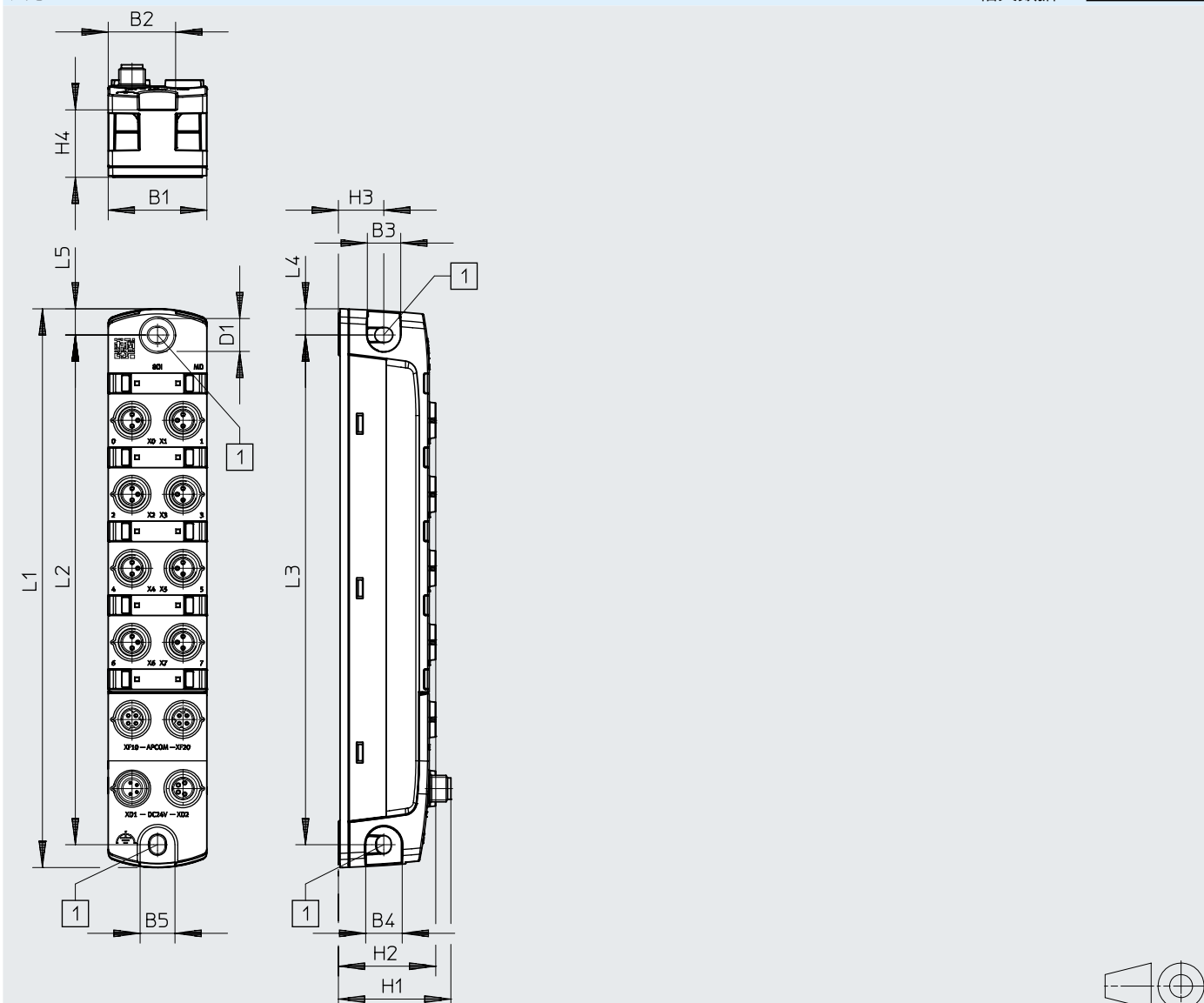
尺寸 - CPX-AP-I-8DI-M8-3P
