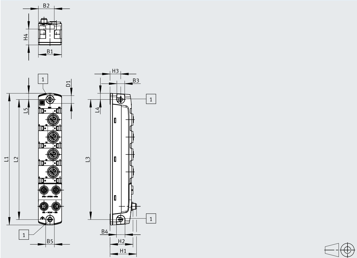
尺寸 – CPX-AP-I-8DO-M12-5P
