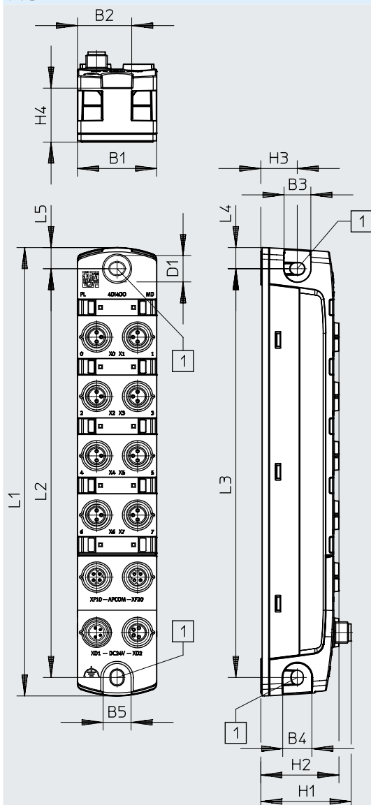
尺寸 – CPX-AP-I-4DI4DO-M8-3P
