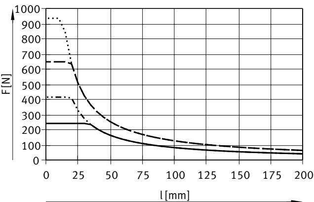
DFM-32 ... 63-KF, 行程最高可达 50 mm
