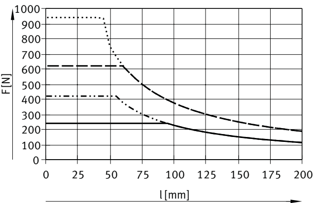
DFM-32 ... 63-GF, 行程 80 ... 100 mm
