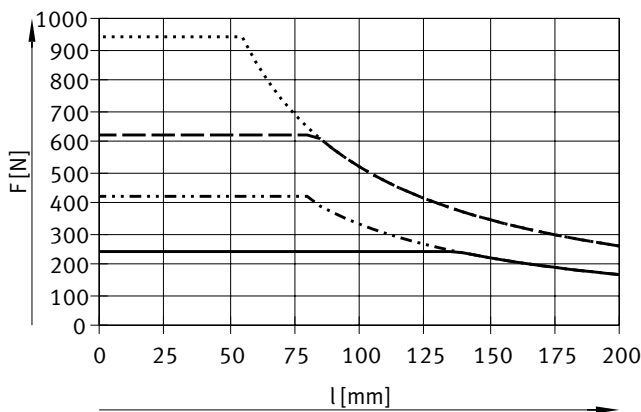
DFM-32 ... 63-GF, 行程 125 ... 200 mm
