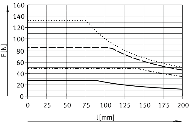
DFM-12 ... 25-KF, 行程 40 ... 100 mm
