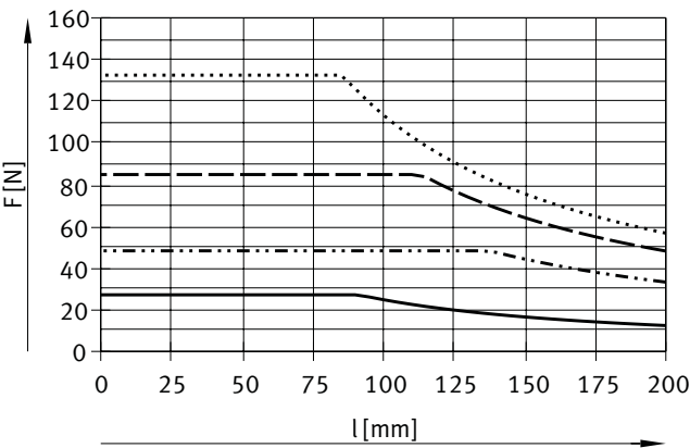
DFM-12 ... 25-GF, 行程 40 ... 100 mm
