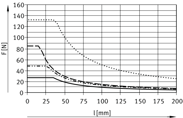
DFM-12 ... 25-GF, 行程最高可达 30 mm
