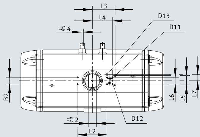
尺寸 - 单作用 DFPD-C, 规格 700 - 2300
