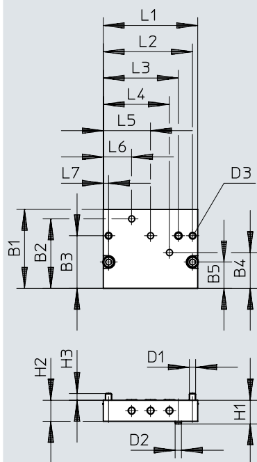
尺寸 – 转接组件 DADG-AK-F9-2
