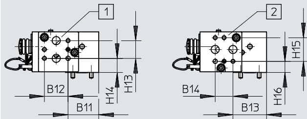
尺寸 – 转接组件 DADG-FM-F9-VDE2
