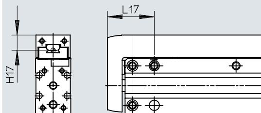
尺寸 - DGSS-...-E1 导轨中心
