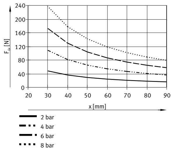
每个夹爪的抓取力 F 与工作压力和杠杆臂 x 的关系 – 外部抓取（合拢），单作用 – DHWC-32-A-S-NO
