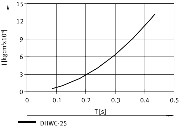
可设置打开和合拢时间 T，在 .6 MPa（6 bar，87 psi）下，与抓手手指的转动惯量的关系 – DHWC-25
