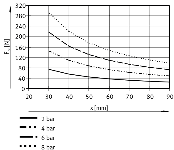
每个夹爪的抓取力 F 与工作压力和杠杆臂 x 的关系 – 内部抓取（打开），双作用 – DHWC-32-A
