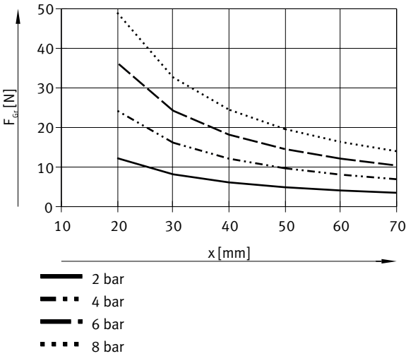
每个夹爪的抓取力 F 与工作压力和杠杆臂 x 的关系 – 内部抓取（打开），双作用 – DHWC-16-A
