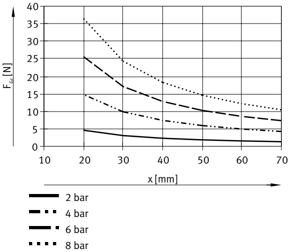
每个夹爪的抓取力 F 与工作压力和杠杆臂 x 的关系 – 外部抓取（合拢），单作用 – DHWC-16-A-S-NO
