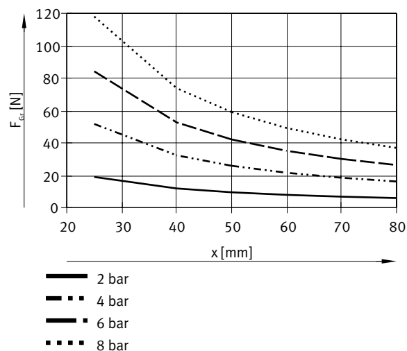
每个夹爪的抓取力 F 与工作压力和杠杆臂 x 的关系 – 外部抓取（合拢），单作用 – DHWC-25-A-S-NO
