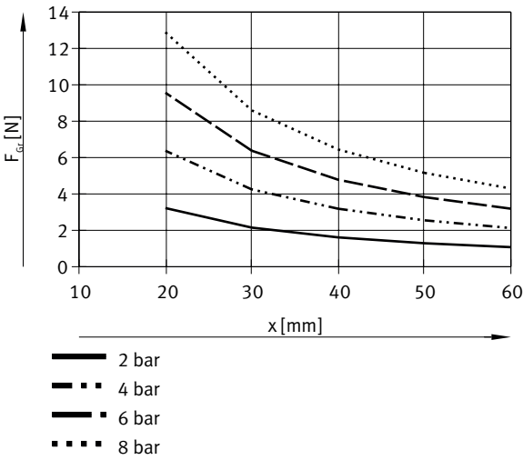
每个夹爪的抓取力 F 与工作压力和杠杆臂 x 的关系 – 外部抓取（合拢），双作用 – DHWC-10-A
