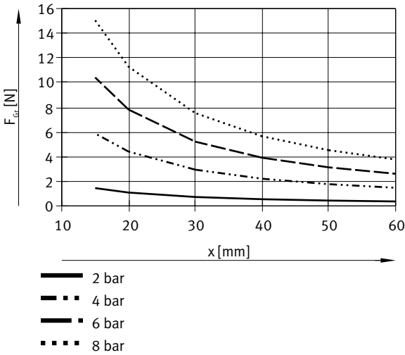
每个夹爪的抓取力 F 与工作压力和杠杆臂 x 的关系 – 外部抓取（合拢），单作用 – DHWC-10-A-S-NO
