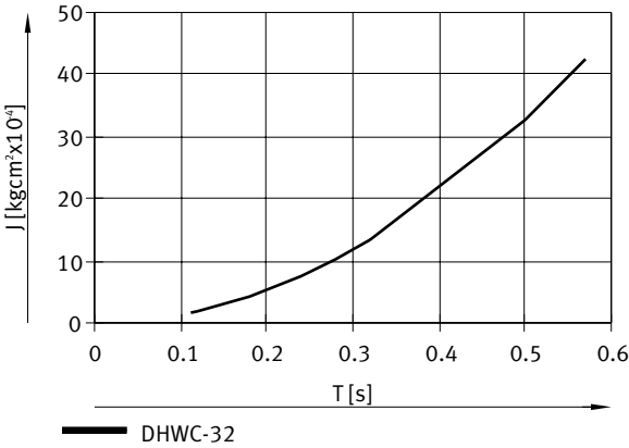
可设置打开和合拢时间 T，在 0.6 MPa（6 bar，87 psi）下，与抓手手指的转动惯量的关系 – DHWC-32
