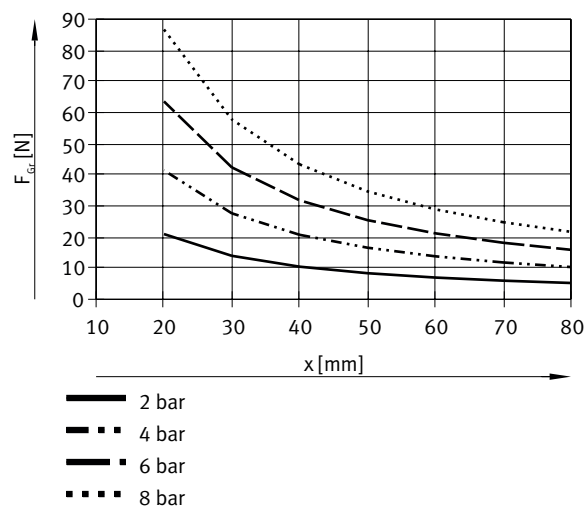
每个夹爪的抓取力 F 与工作压力和杠杆臂 x 的关系 – 外部抓取（合拢），双作用 – DHWC-20-A
