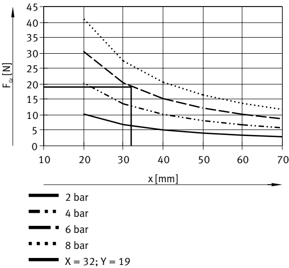
在 0.6 MPa (6 bar, 87 psi) 下每个夹爪的抓取力 F 与杠杆臂 x 及偏心率 a 和 b 的关系
