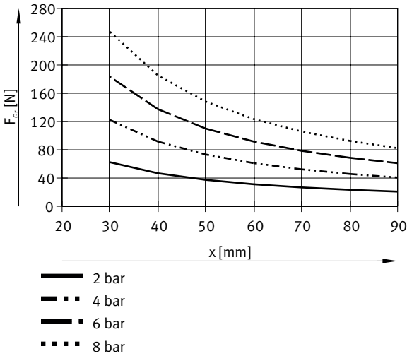
每个夹爪的抓取力 F 与工作压力和杠杆臂 x 的关系 – 外部抓取（合拢），双作用 – DHWC-32-A
