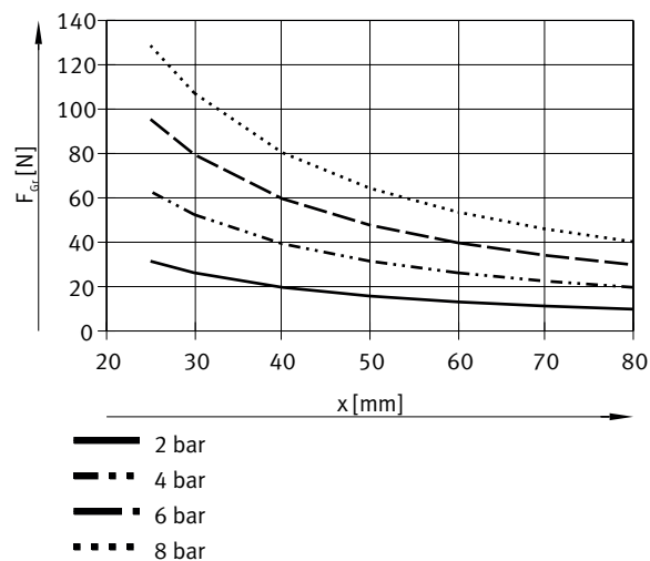
每个夹爪的抓取力 F 与工作压力和杠杆臂 x 的关系 – 外部抓取（合拢），双作用 – DHWC-25-A
