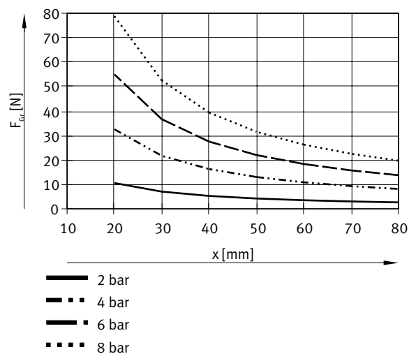
每个夹爪的抓取力 F 与工作压力和杠杆臂 x 的关系 – 外部抓取（合拢），单作用 – DHWC-20-A-S-NO
