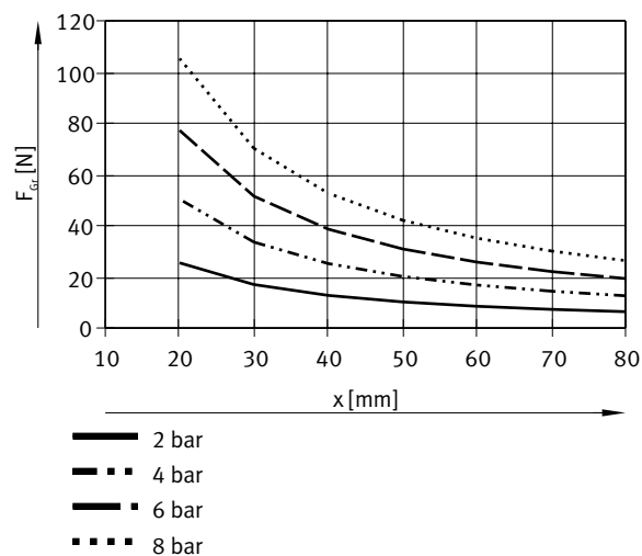
每个夹爪的抓取力 F 与工作压力和杠杆臂 x 的关系 – 内部抓取（打开），双作用 – DHWC-20-A
