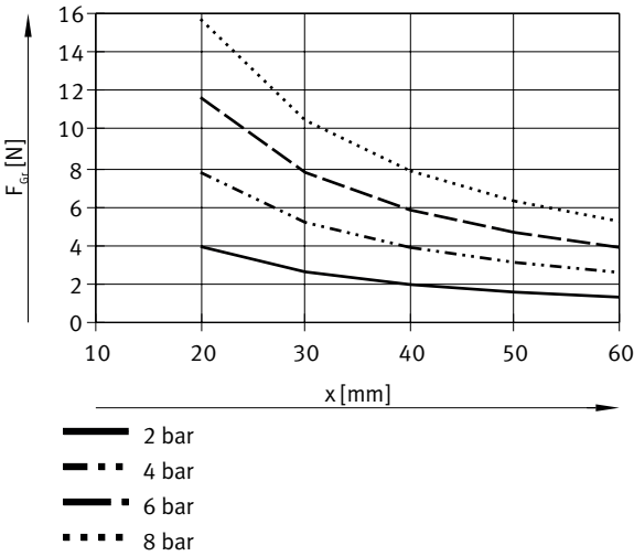
每个夹爪的抓取力 F 与工作压力和杠杆臂 x 的关系 – 内部抓取（打开），双作用 – DHWC-10-A
