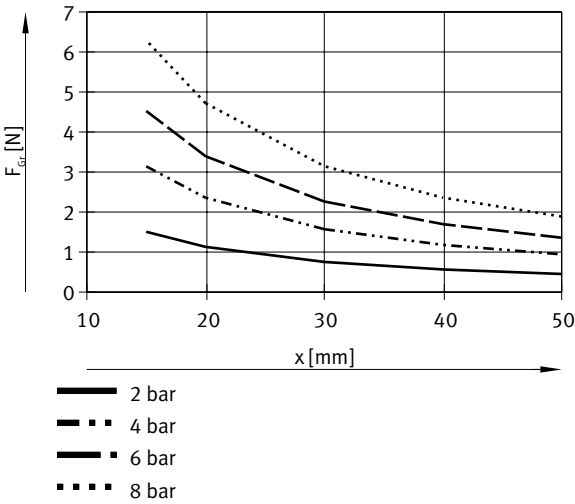
每个夹爪的抓取力 F 与工作压力和杠杆臂 x 的关系 – 内部抓取（打开），双作用 – DHWC-6-A
