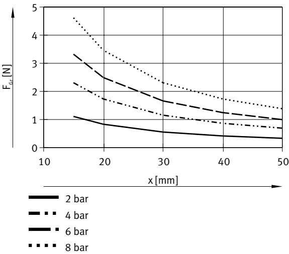
每个夹爪的抓取力 F 与工作压力和杠杆臂 x 的关系 – 外部抓取（合拢），双作用 – DHWC-6-A
