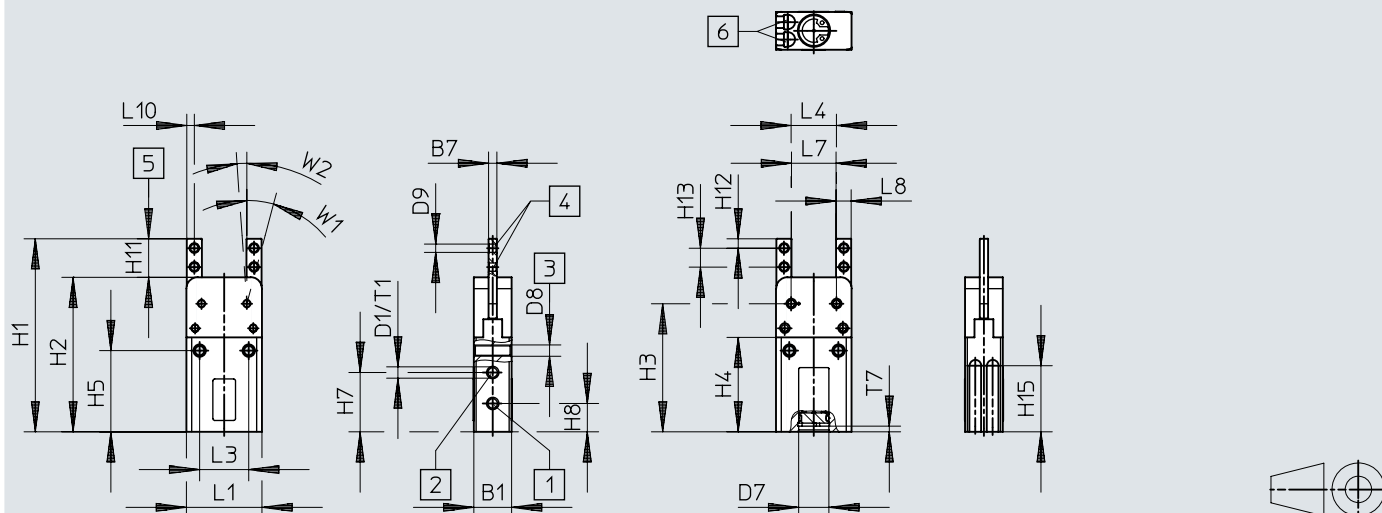
尺寸 - DHWC-6
