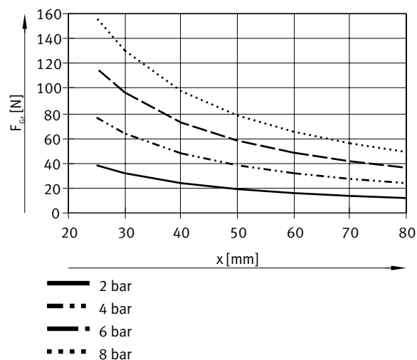
每个夹爪的抓取力 F 与工作压力和杠杆臂 x 的关系 – 内部抓取（打开），双作用 – DHWC-25-A
