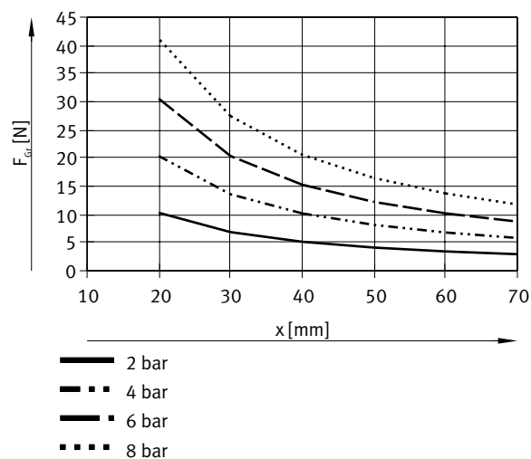
每个夹爪的抓取力 F 与工作压力和杠杆臂 x 的关系 – 外部抓取（合拢），双作用 – DHWC-16-A
