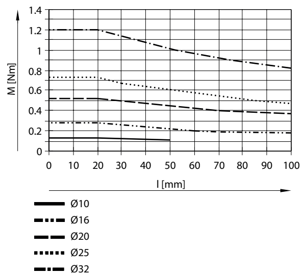
许用扭矩 M 与行程 L 的关系 - 双端活塞杆 - 循环滚珠轴承导轨
