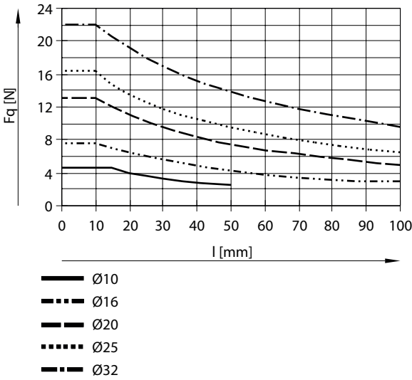
许用横向负载 F 与行程 L 的关系 - 一端活塞杆 - 循环滚珠轴承导轨
