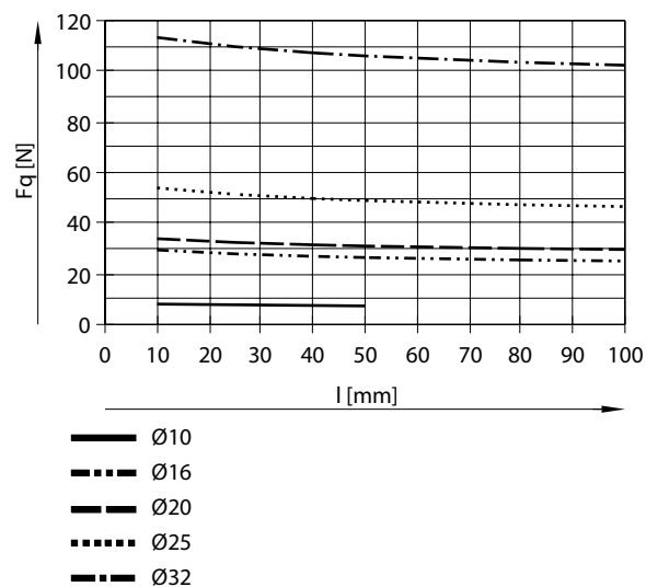
许用横向负载 F 与行程 L 的关系 - 双端活塞杆 - 滑动轴承导轨
