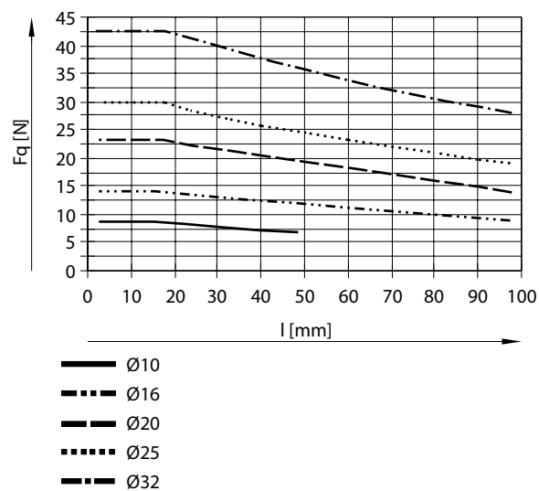
许用横向负载 F 与行程 L 的关系 - 双端活塞杆 - 循环滚珠轴承导轨
