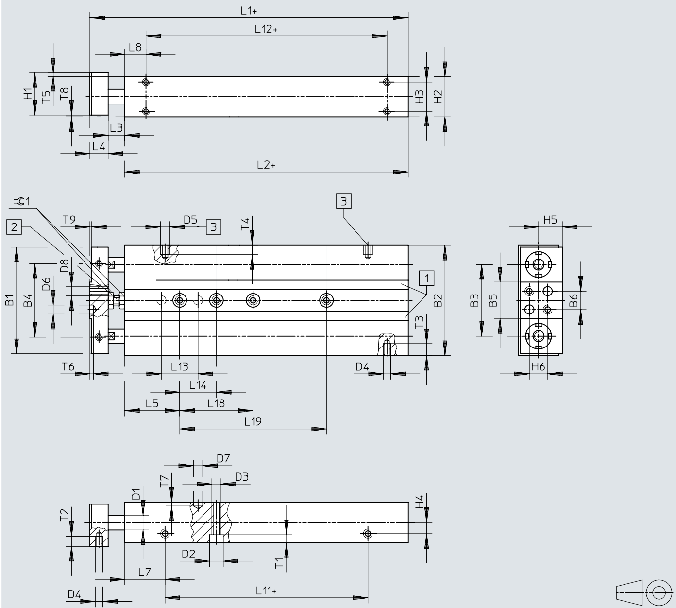
尺寸 - DPZ-10/-16 - 带端板
