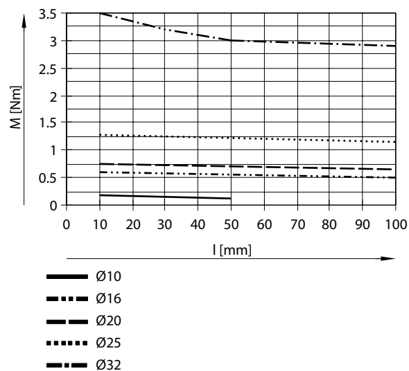
许用扭矩 M 与行程 L 的关系 - 双端活塞杆 - 滑动轴承导轨
