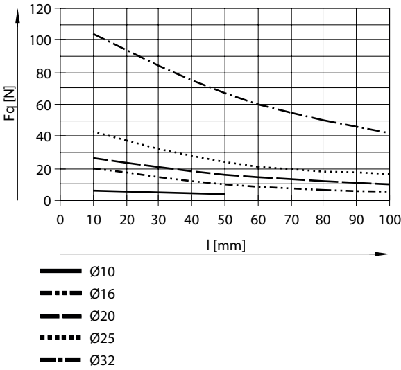
许用横向力 F 与行程 L 的关系 - 一端活塞杆 - 滑动轴承导轨
