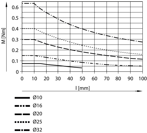
许用扭矩 M 与行程 L 的关系 - 一端活塞杆 - 循环滚珠轴承导轨
