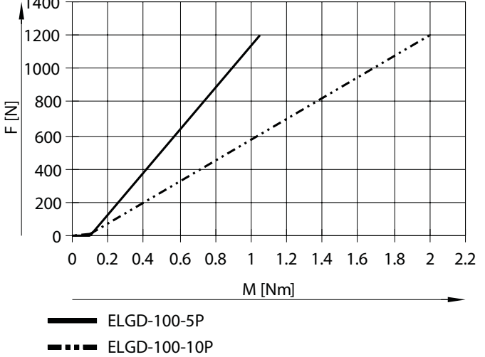
进给力 F 与输入扭矩 M 的关系
