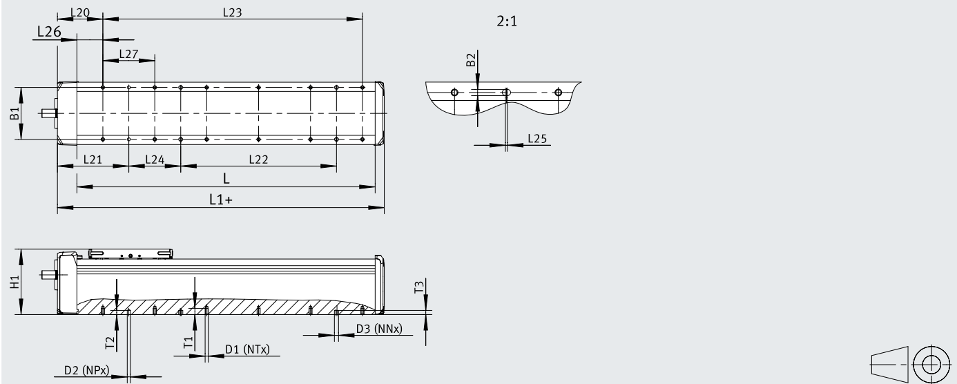
尺寸 – ELGD-BS-...-M (用于直接安装)
