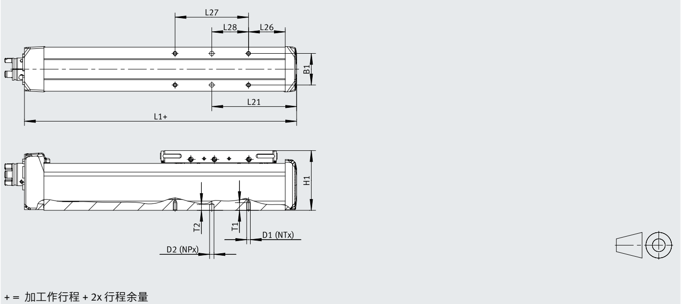
尺寸 – ELGD-BS-...-M7 (用于正面安装)
