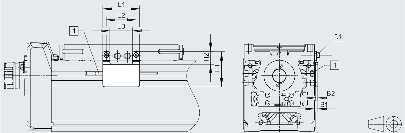
尺寸 - 传感器感应片 EAPM-E24-60-SLS
