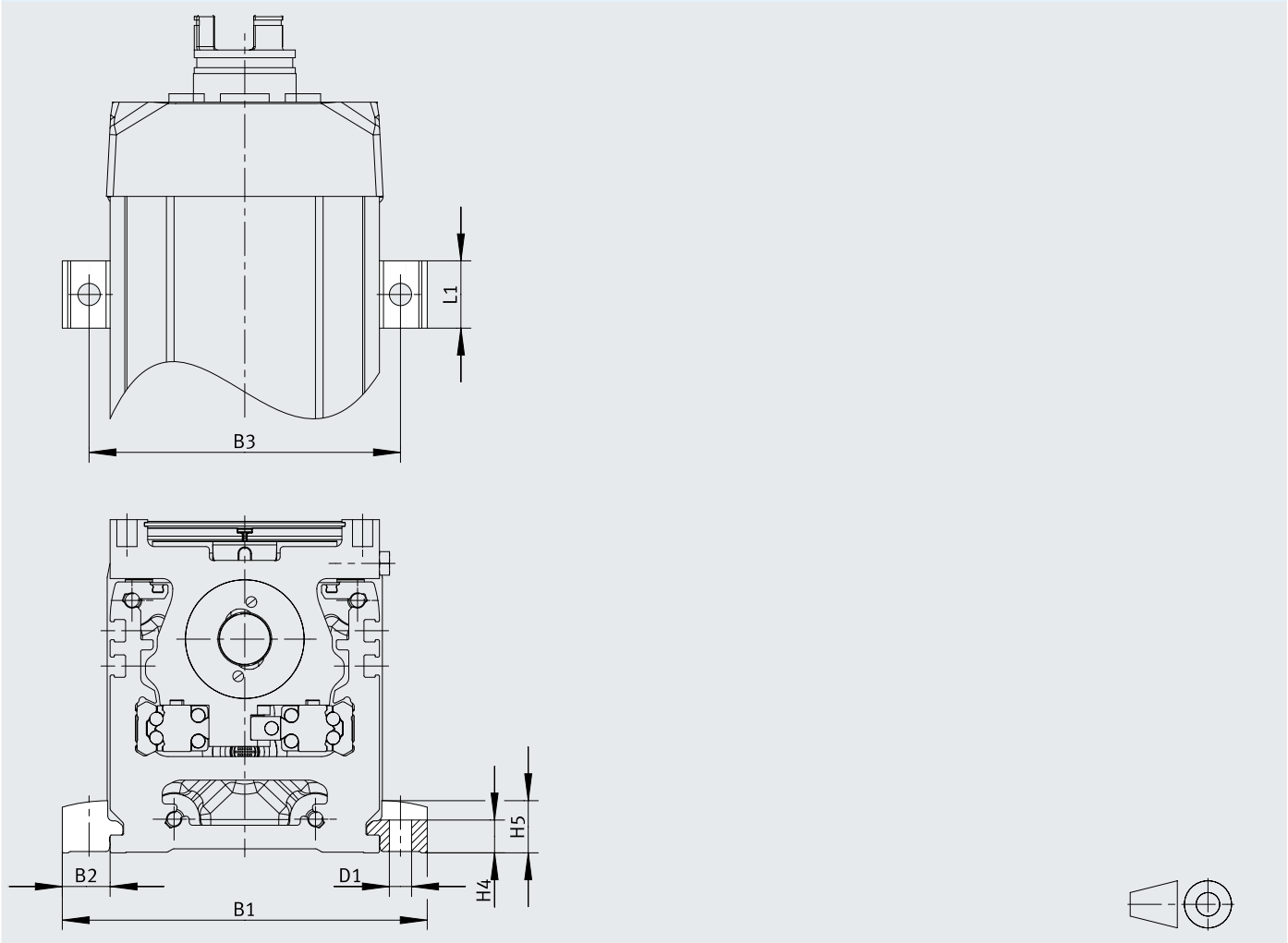
尺寸 - 型材安装件 EAHF-E24-60-P-S
