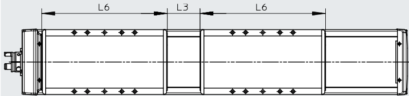
尺寸 – ELGD-BS-...-ZR (带附加滑块)
