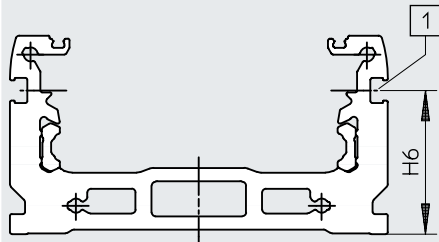
尺寸 – ELGD-BS-...- (型材)
