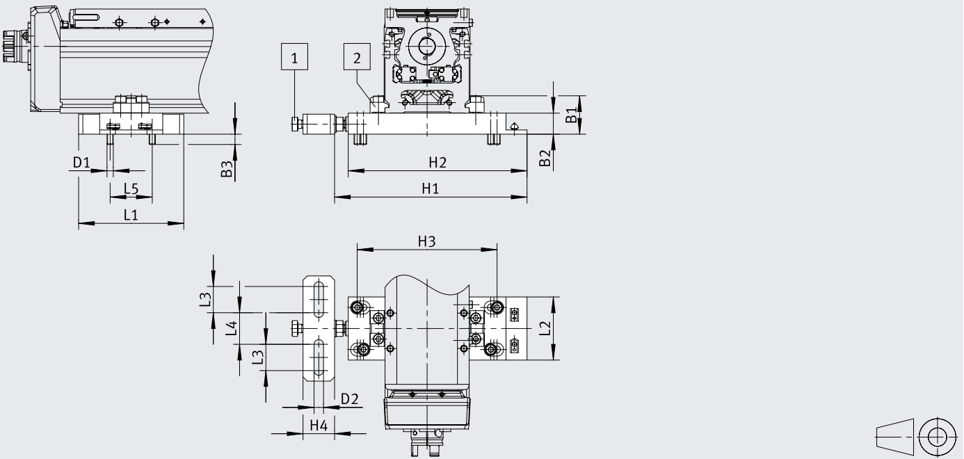
尺寸 - 调节组件 EADC-E16-...
