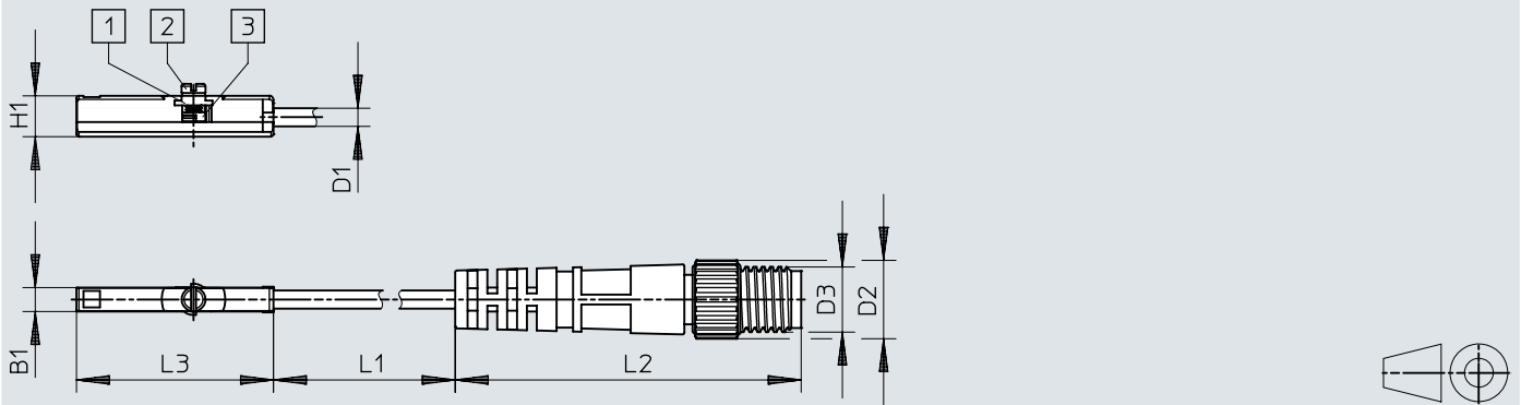
尺寸 – 接近开关，带插头
