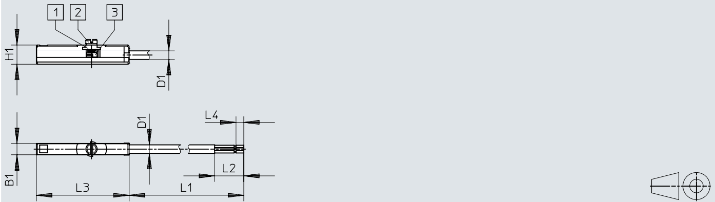
尺寸 – 带开放端部的接近开关 SDBC-MSB-1L-PU/NU-...
