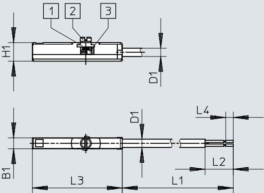
尺寸 – 带开放端部的接近开关 SDBC-MSB-1L-ZU-...
