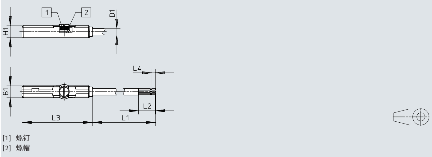
尺寸 – 开放式接近开关 SDBT-MSB-1L-PU/NU-...
