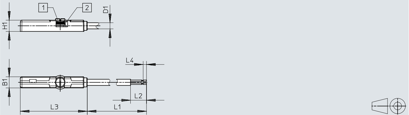
尺寸 – 接近开关，开放式，SDBT-MSB-1L-ZU-...
