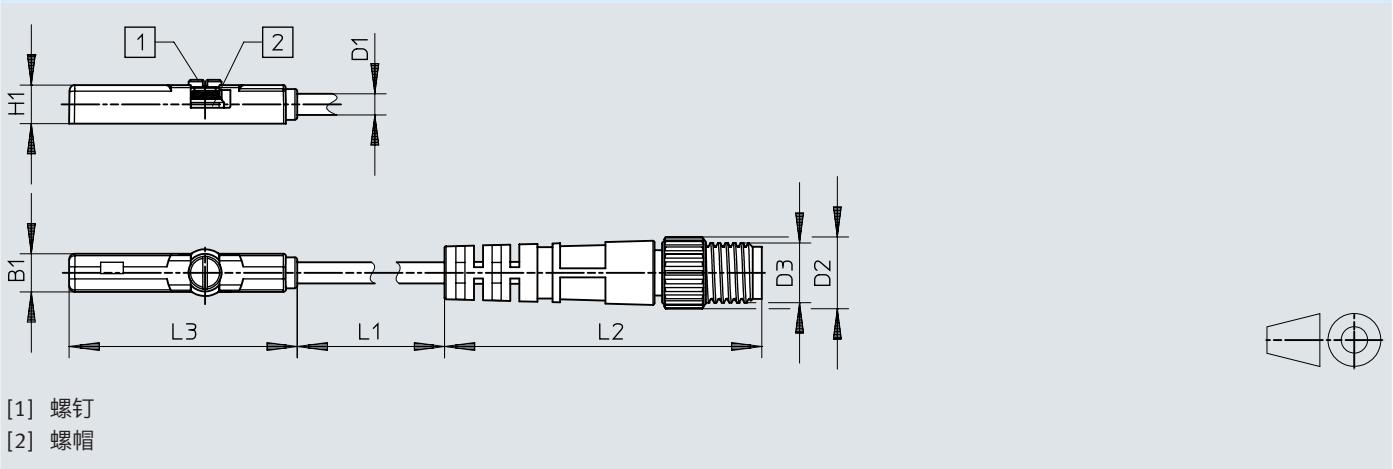
尺寸 – 接近开关，带插头
