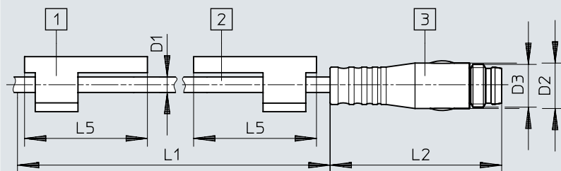
尺寸 - M8 - 电缆, 带插头 M8x1, 卡环
