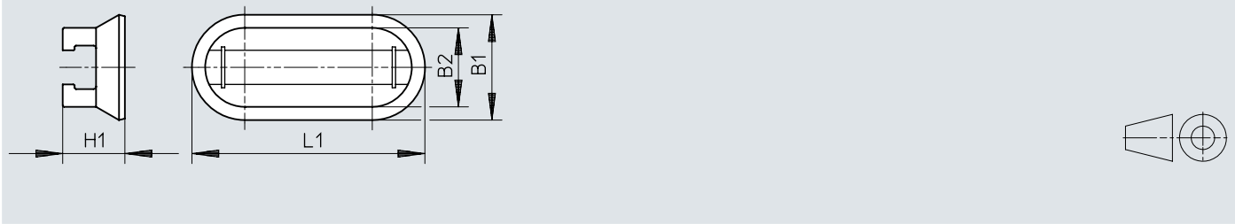
尺寸 – 安装组件 CRSMB
