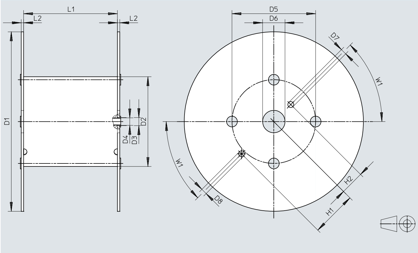
尺寸 - 辊筒
