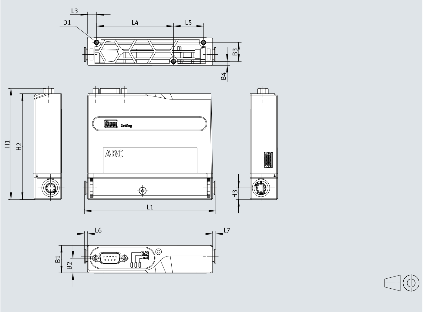
尺寸 – 质量流量控制器 VEFC, Q8
