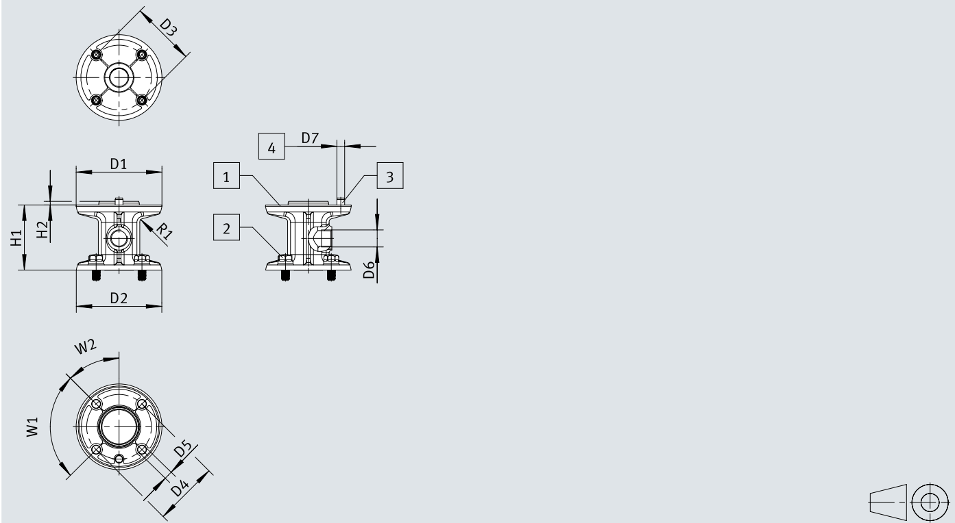
尺寸 – 转接组件 HAMA-MA-B33-RA50
