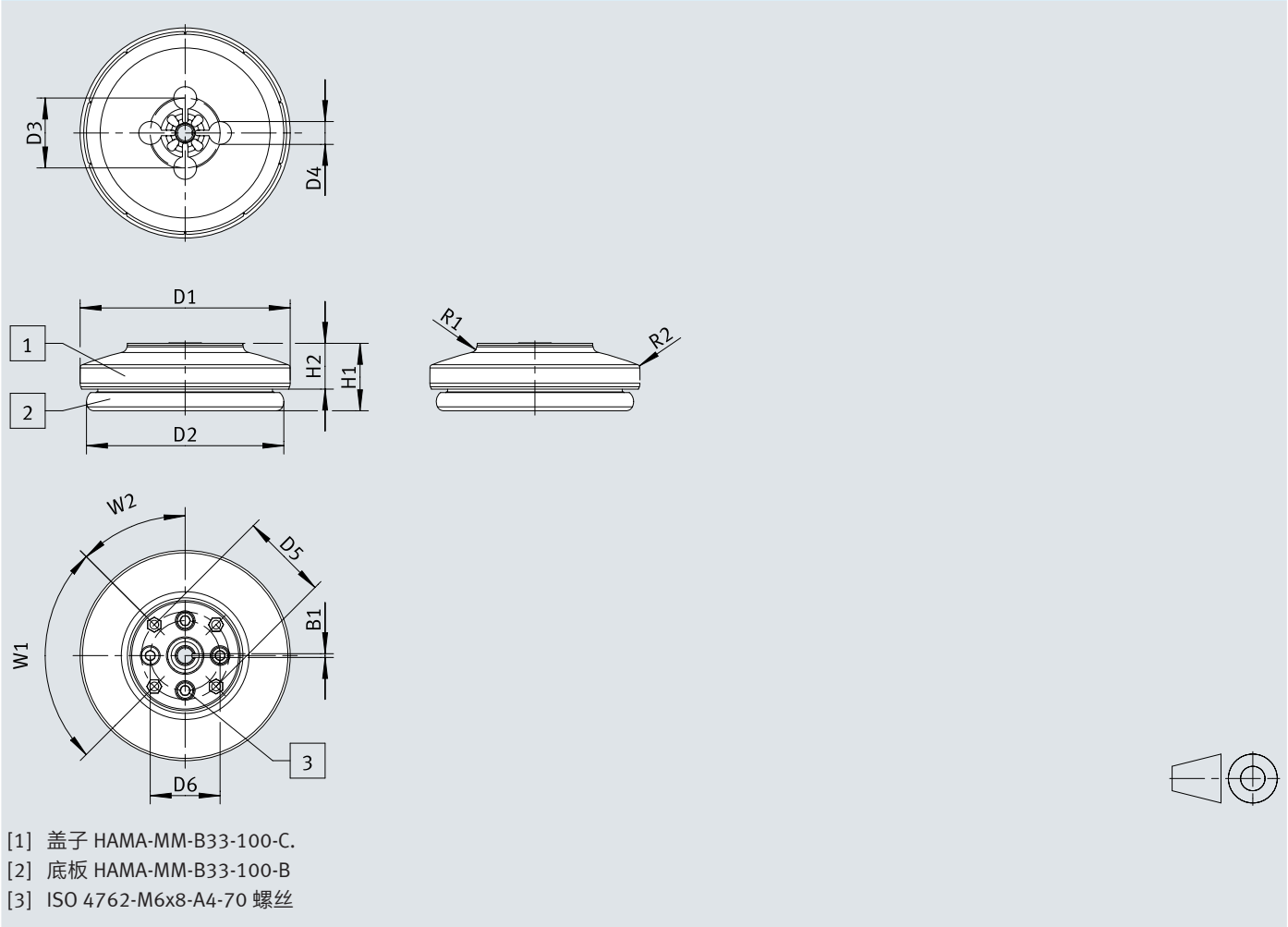
尺寸 – 安装组件 HAMA-MM-B33-100
