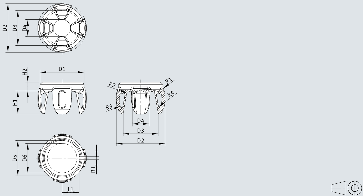
尺寸 – 手指本体 HAMA-GA-B33-70-4-S-40-BU
