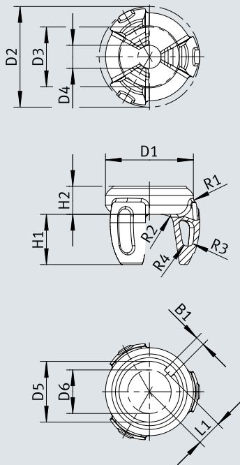
尺寸 - 手指本体 HAMA-GA-B33-40-3-S-40-BU
