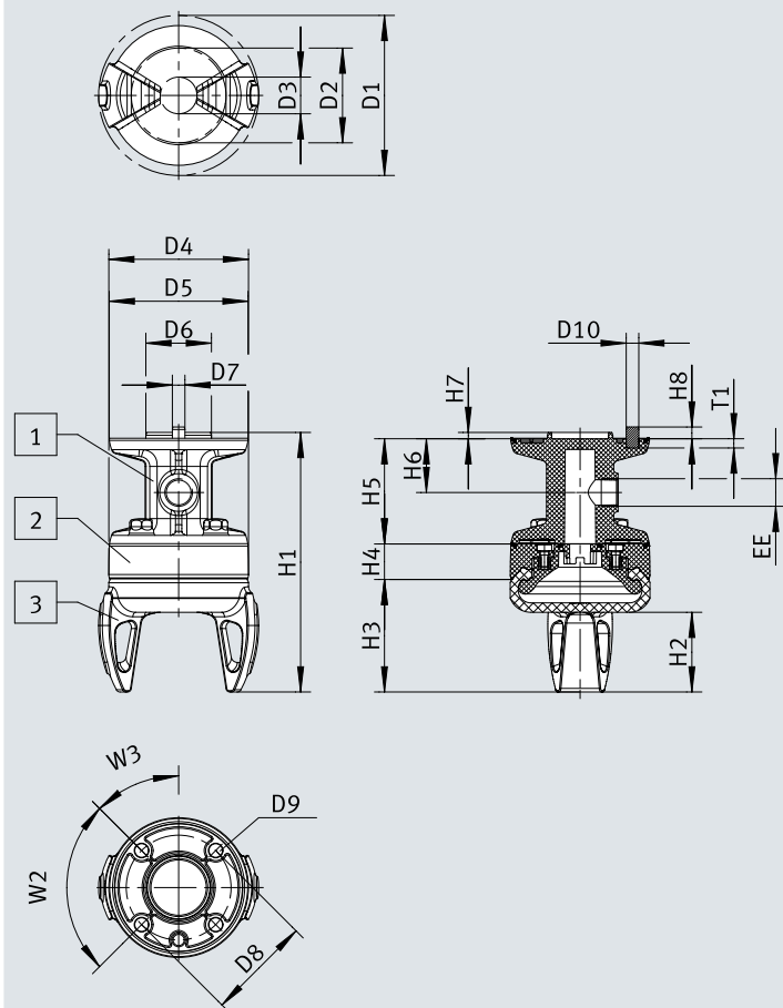
尺寸 – HPSX 软手指，配备 2 手指
