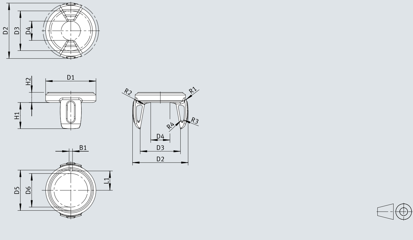
尺寸 - 手指本体 HAMA-GA-B33-70-2-S-40-BU
