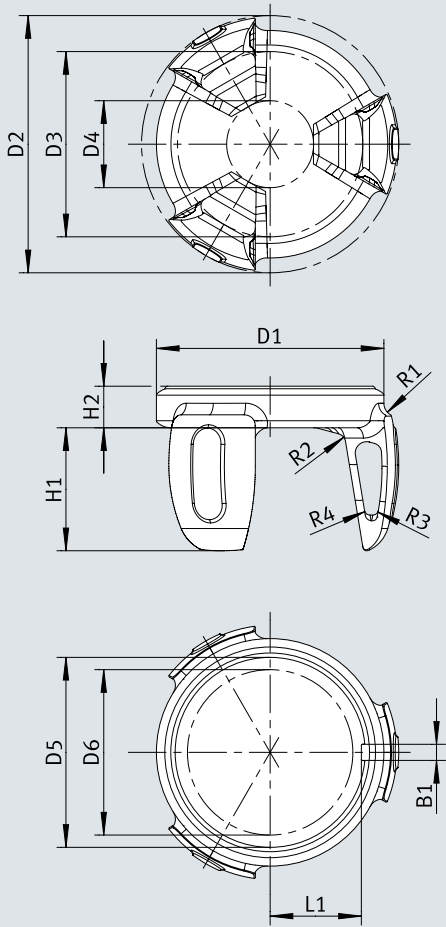
尺寸 - 手指本体 HAMA-GA-B33-100-3-S-40-BU
