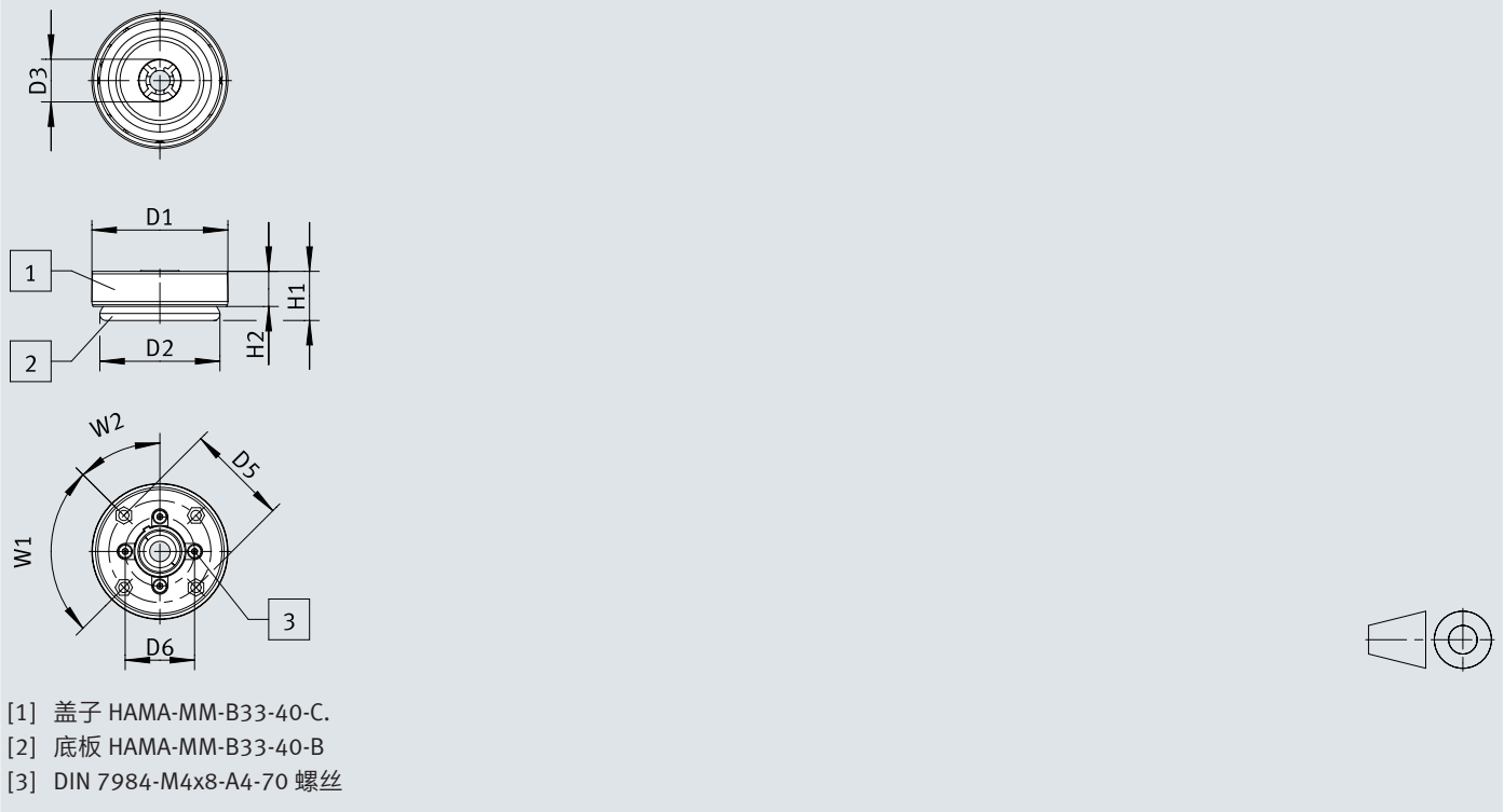
尺寸 – 安装组件 HAMA-MM-B33-40
