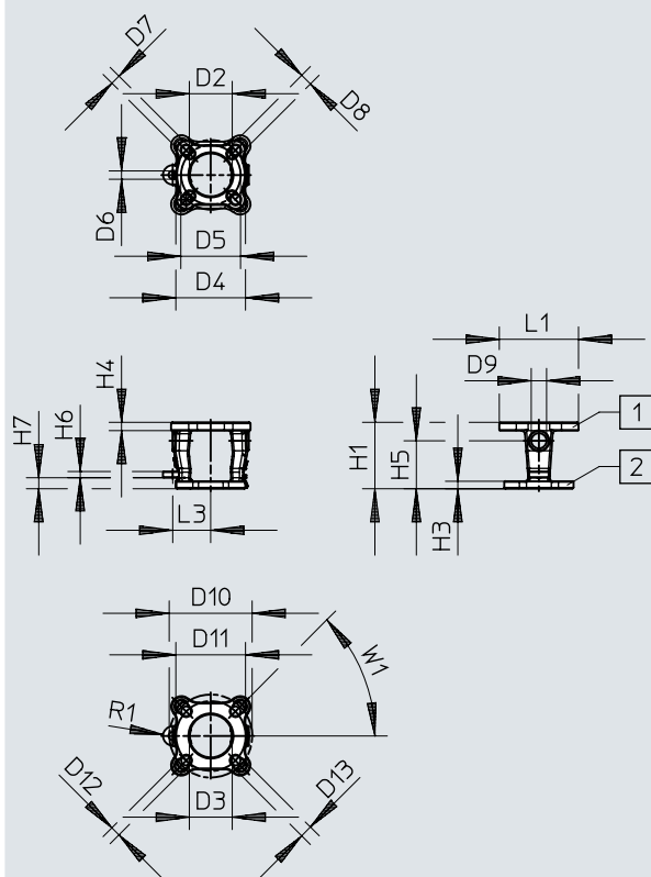
尺寸 – 安装连接件 DARQ-B-...R1
