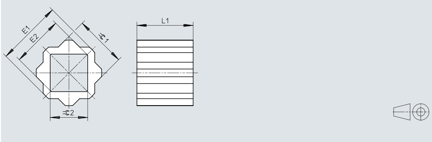
尺寸 – 变径轴套 DARQ
