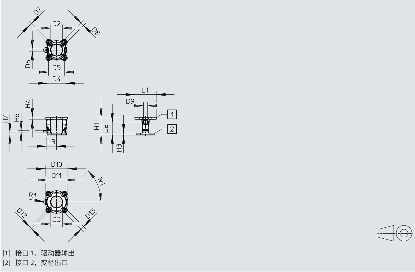
尺寸 – 安装转接件 DARQ-B-...R1
