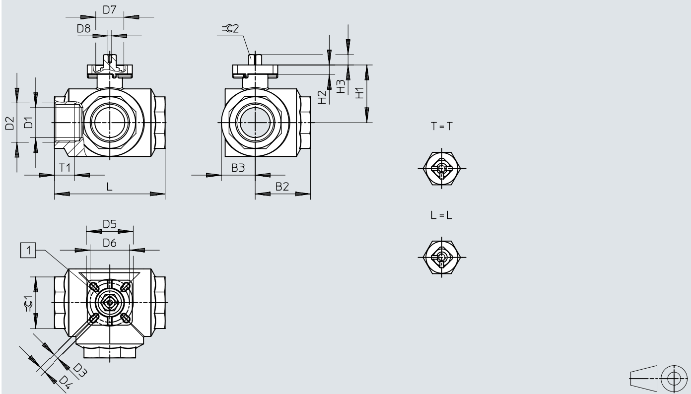
尺寸 – 三通球阀 VZBM
