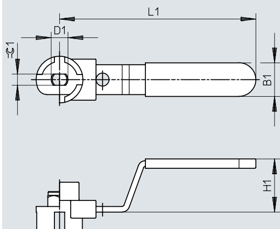
尺寸 - 手动手柄 VAOH
