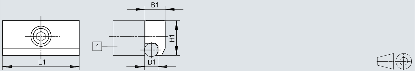
尺寸 – 安装组件 SMB-1
