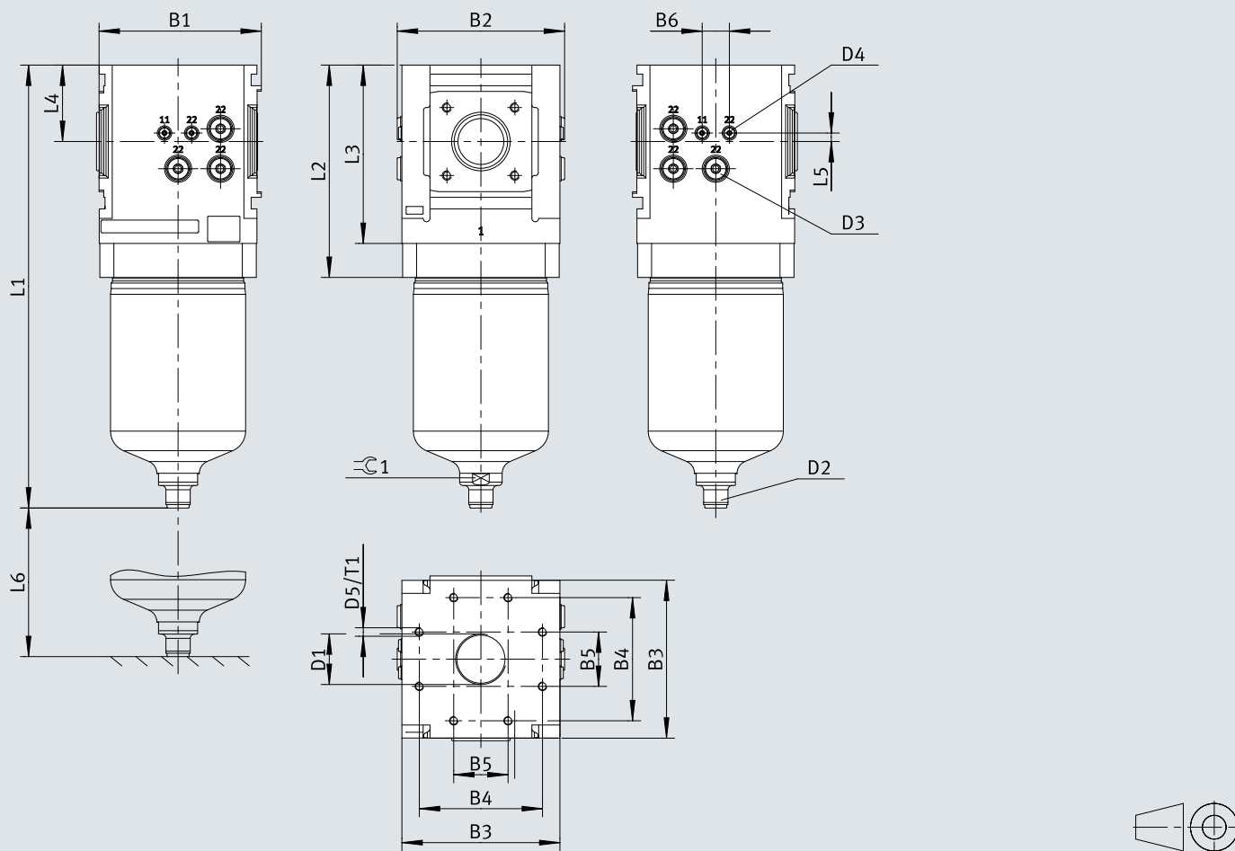
尺寸 - PFML-186-HP3-H-AST
