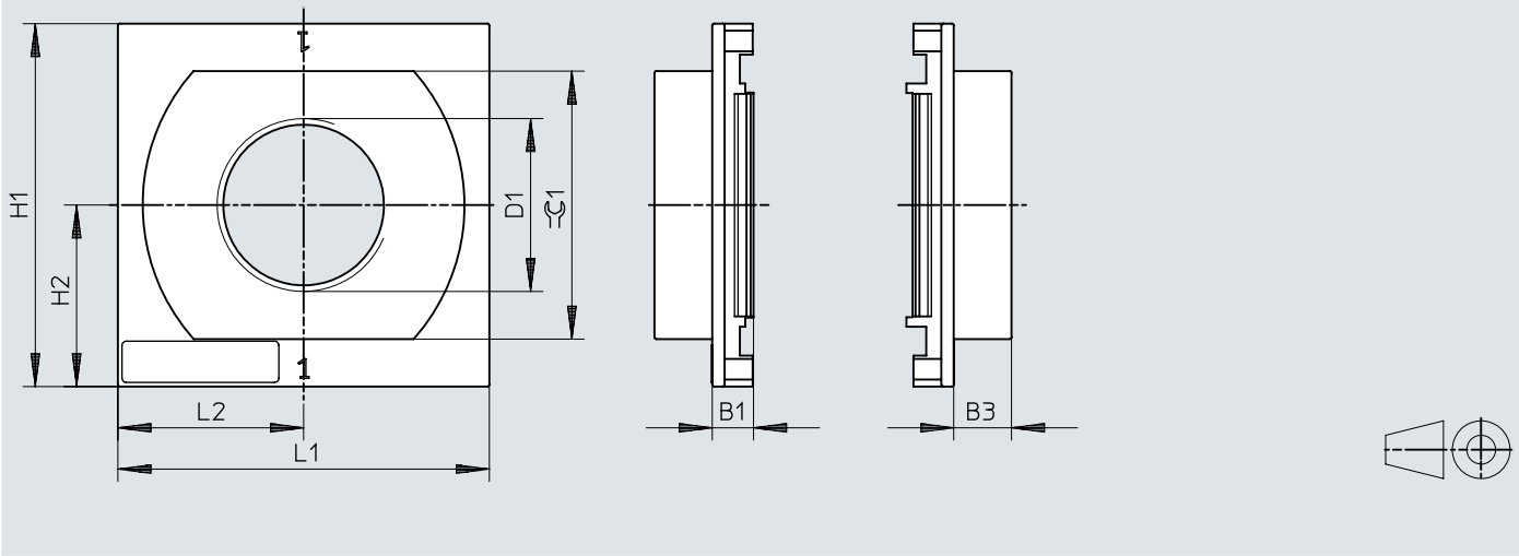
尺寸 – 连接板 PAML-CP-90-HP3-G114
