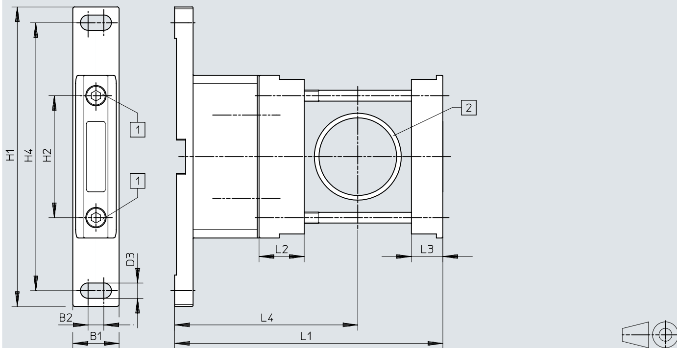
尺寸 - 安装支架 PAML-MB
