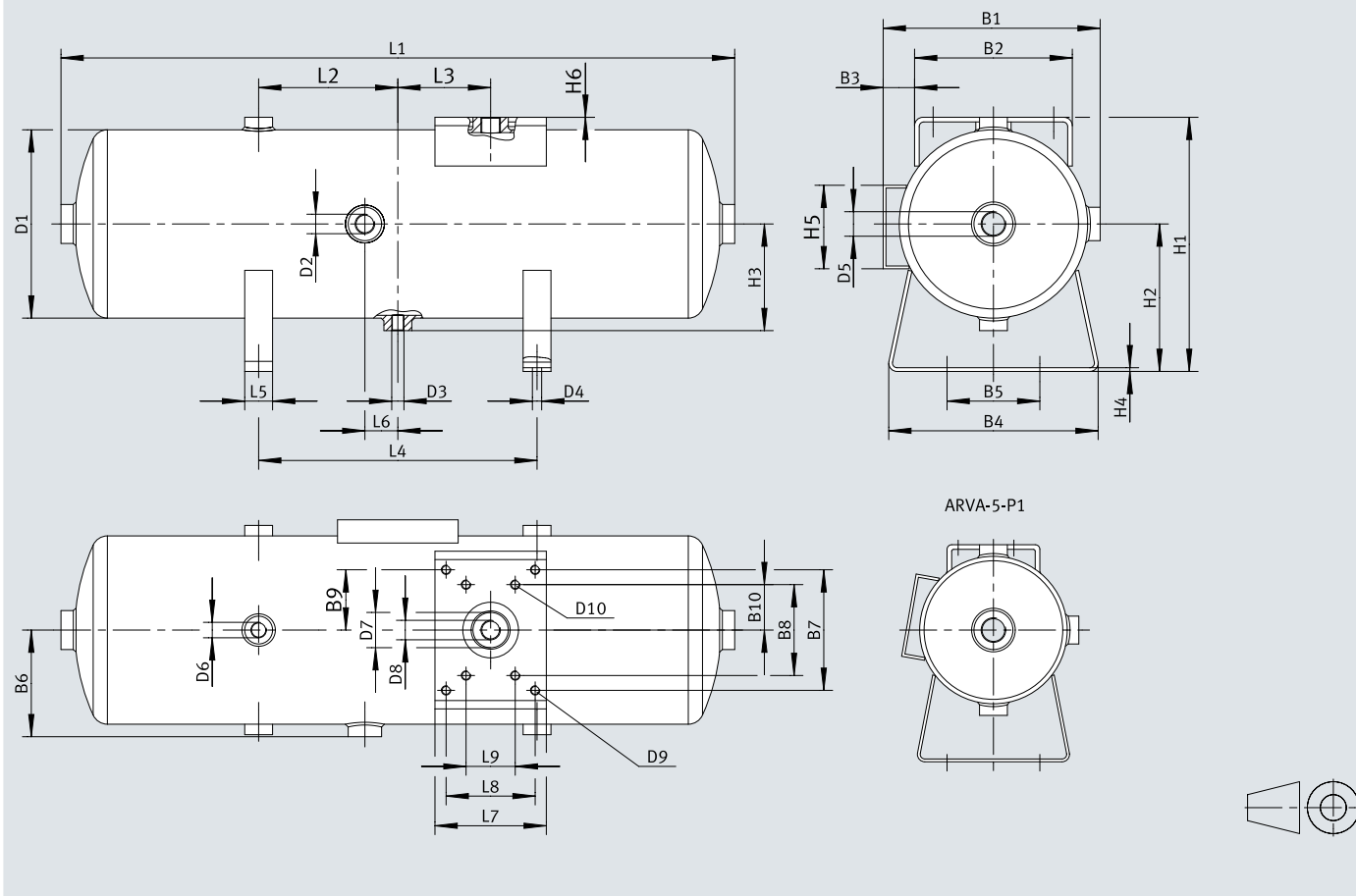
尺寸 - ARVA-...-P1
