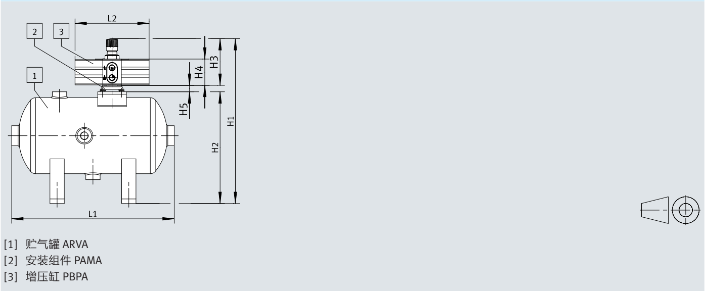
尺寸 – ARVA-...-P1, 带增压缸 PBPA
