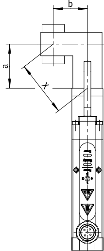
抓取力 F 与杠杆臂 x 及偏心率 a 和 b 的关系
