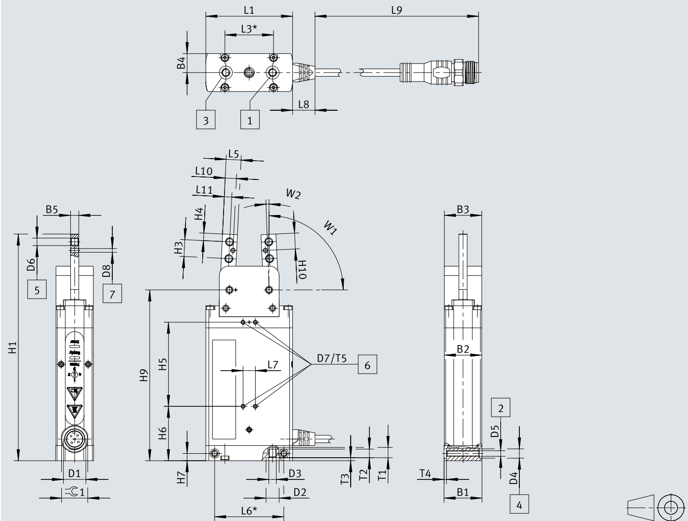
尺寸 - 旋转抓手 HERC
